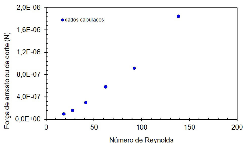
Figura 10. Relação entre força de arrasto ou de corte e o número de Reynolds.
